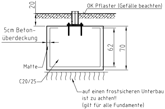
Schnitt A-A
